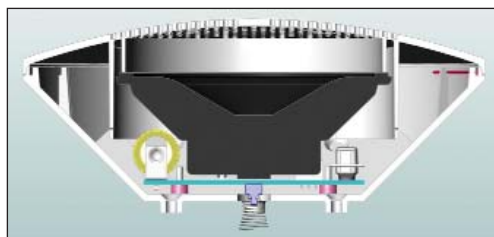
Рис.3 Датчик отрыва от строительных конструкций
