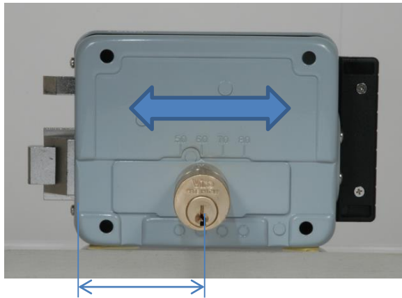
Регулируемый выход от 50 до 80 mm
